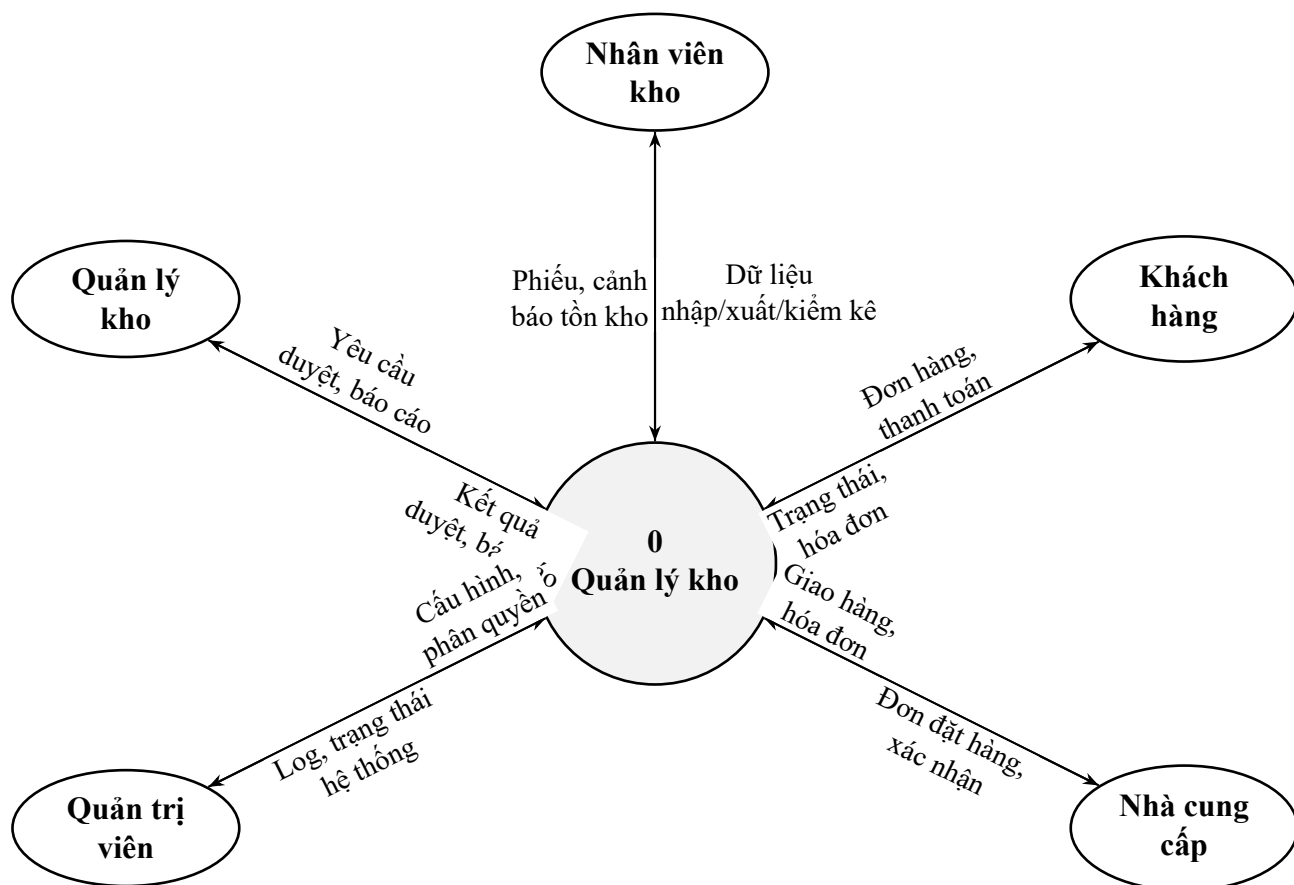
Hình 1: DFD cấp 0 (Context Diagram) – Hệ thống quản lý kho hàng
